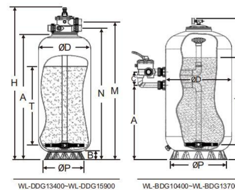
WL-BDG10400-WL-BDG13700
