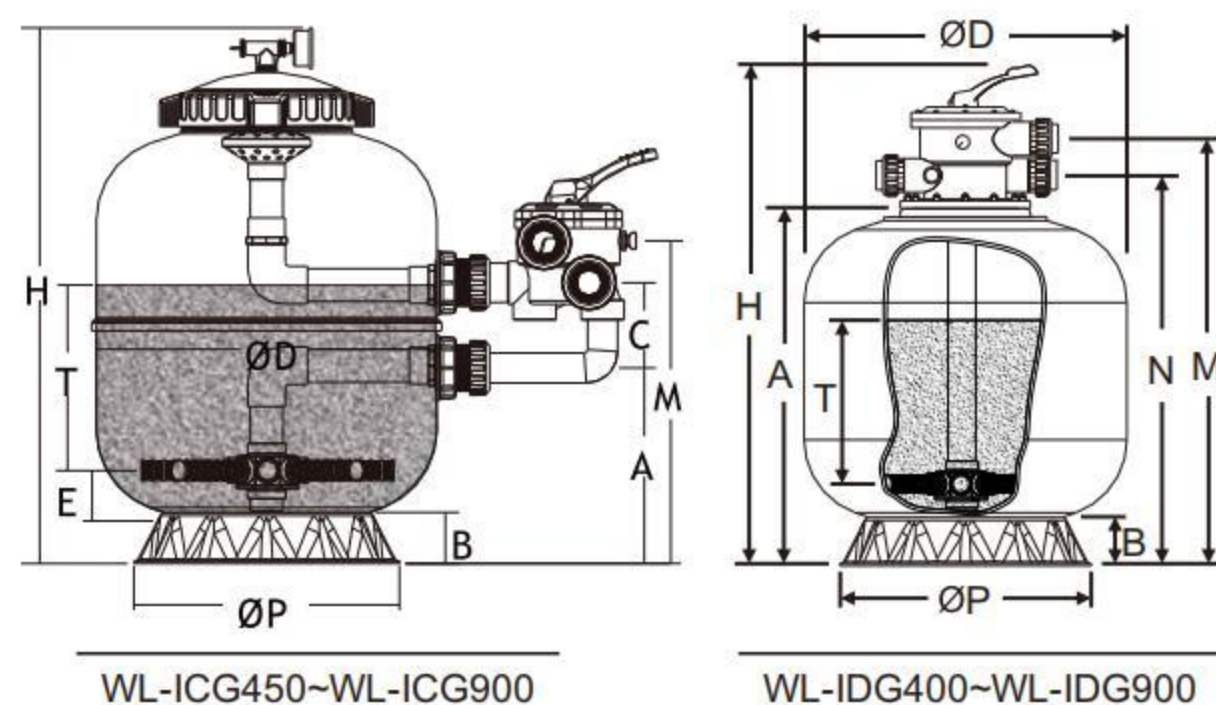
WL-ICG450~WL-ICG900
